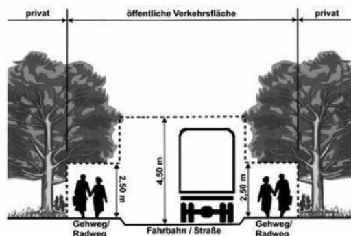
Skizze zum Freischneiden des lichten Verkehrsraumprofils
