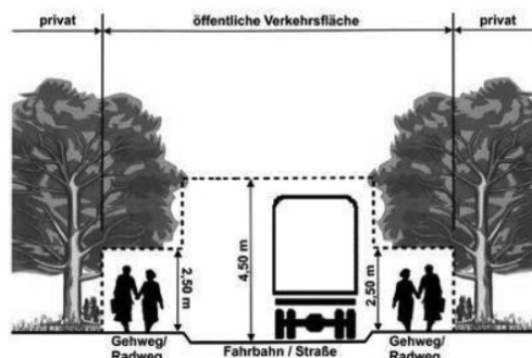
Skizze zum Freischneiden des lichten Verkehrsraumprofils
